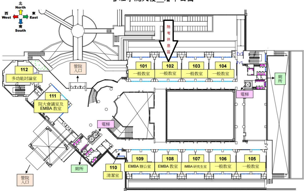
管理學院大樓一層平面圖
